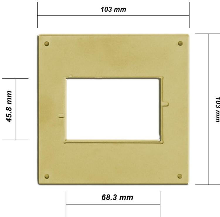
安装视图 01
