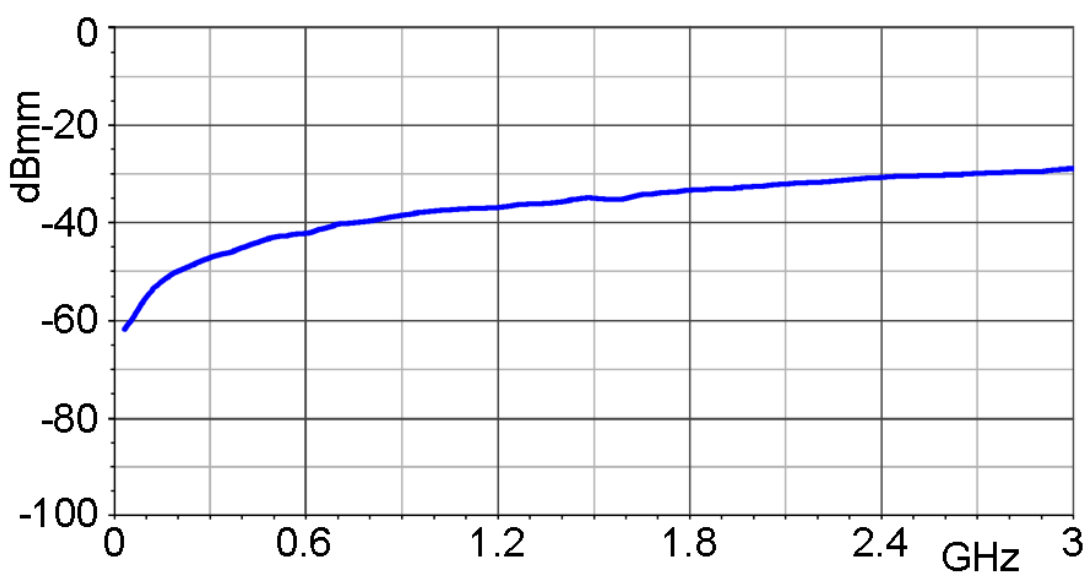
频率特性
