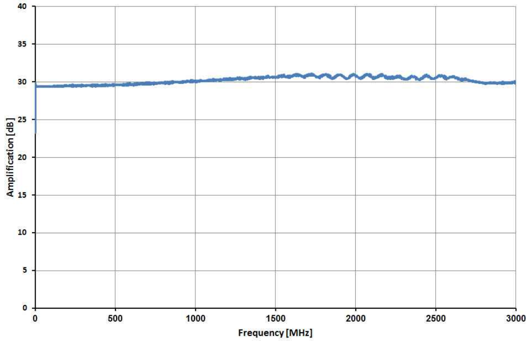
频率特性
